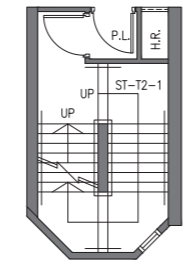
第2座(2B) 30樓至36樓 部份平面圖 PART PLAN AT 30/F TO 36/F OF TOWER 2 (2B)
