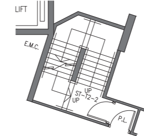
第2座(2A) 30樓至36樓 部份樓平面圖 PART PLAN AT 30/F TO 36/F OF TOWER 2 (2A)
